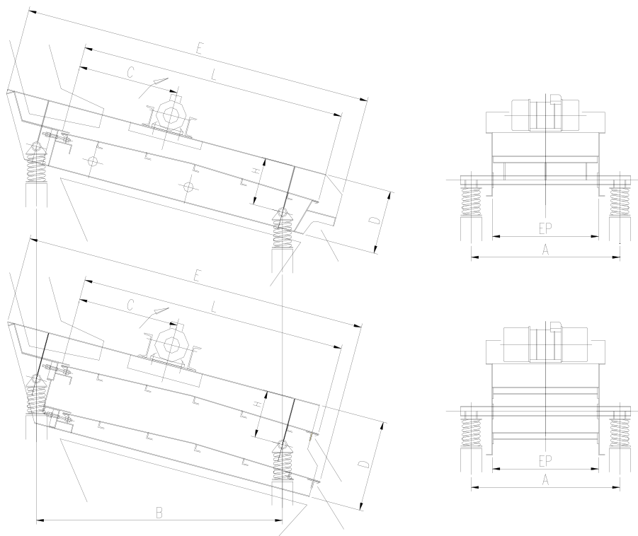
DIMENSIONS GENERALES DES CRIBLES INCLINES A MOTOVIBRATEURS (mm)
