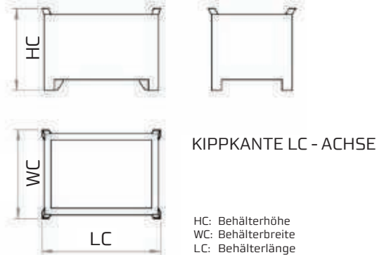
BEHÄLTERABMESSUNGEN
