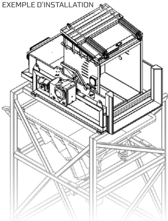
EXEMPLE D'INSTALLATION
