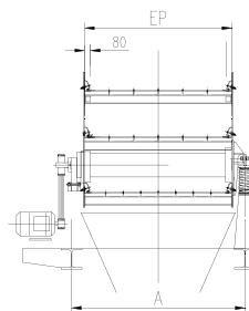
KEILRIEMEN-ANTRIEB
