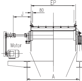
ENTRAÎNEMENT PAR PALIER INTERMÉDIAIRE
