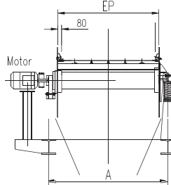
DIMENSIONS GÉNÉRALES (mm)
