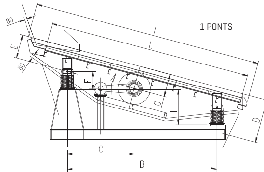
ENTRAÎNEMENT PAR SYSTÈME POULIE/COURROIE
