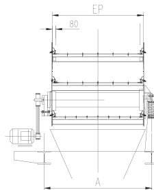
ENTRAINEMENT PAR SYSTEME POULIE/COURROIE
