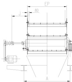
ENTRAINEMENT PAR PALIER INTERMEDIAIRE
