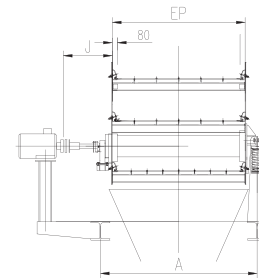
ENTRAINEMENT DIRECT
